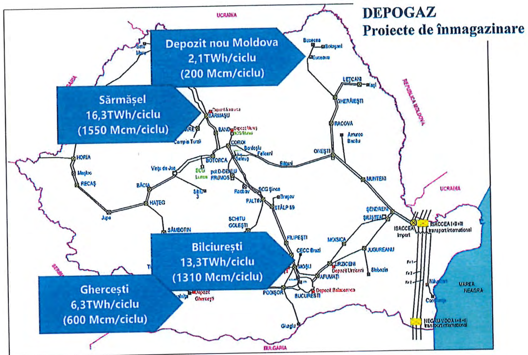
Figura 25 – Proiecte majore de înmagazinare gaze naturale – Depogaz
